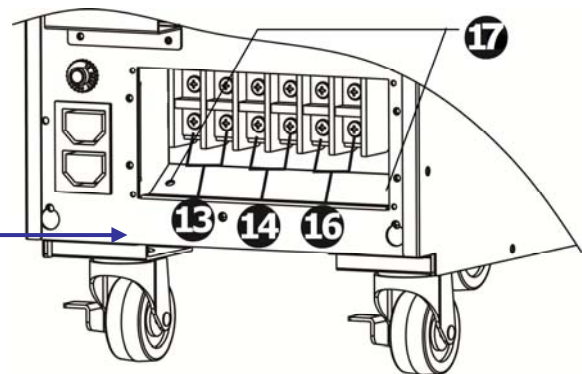
Figura 2: Conexión entrada/salida
